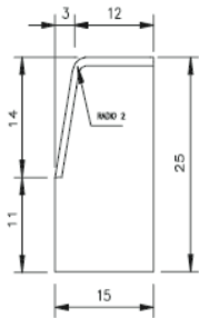
BORDILLO DE CALZADA C5
